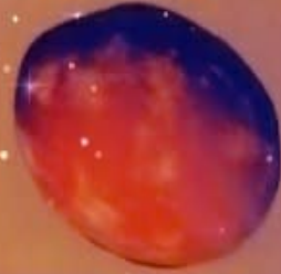
Mars
