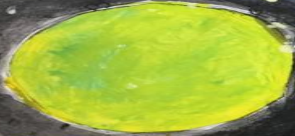
المريخ .
