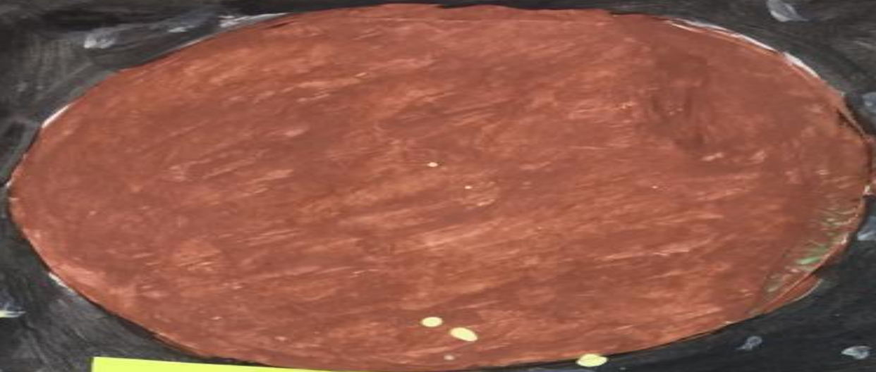
اورانوس .
