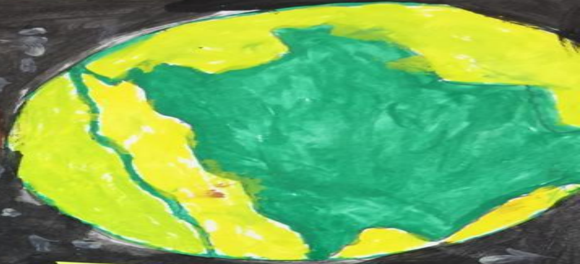
الارض .
