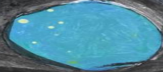
القمر .
